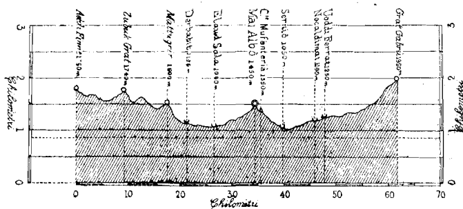
FIG. 10 a . — Profilo altimetrico da Grati Gabrù a Addi Finni.
