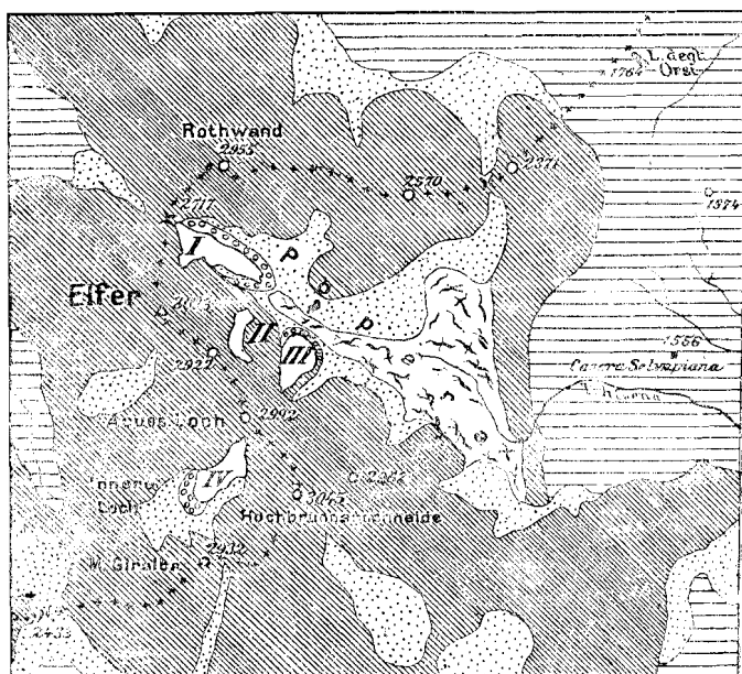
FIG. 16 A . — Schizzo morfologico del gruppo dell'Elfer nelle Alpi di Sesto.
