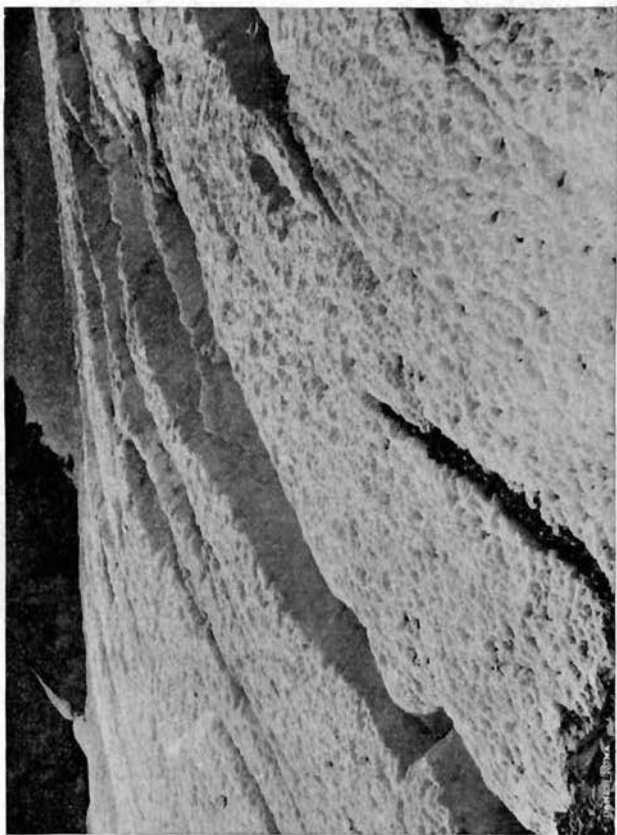
FIG. 15 a . — Area crepacciata nel ghiacciaio del Këllervand. (Da una fotografia del signor A. Ferrucci, presa il 1° settembre 1900, dal nasso col segno I°).
