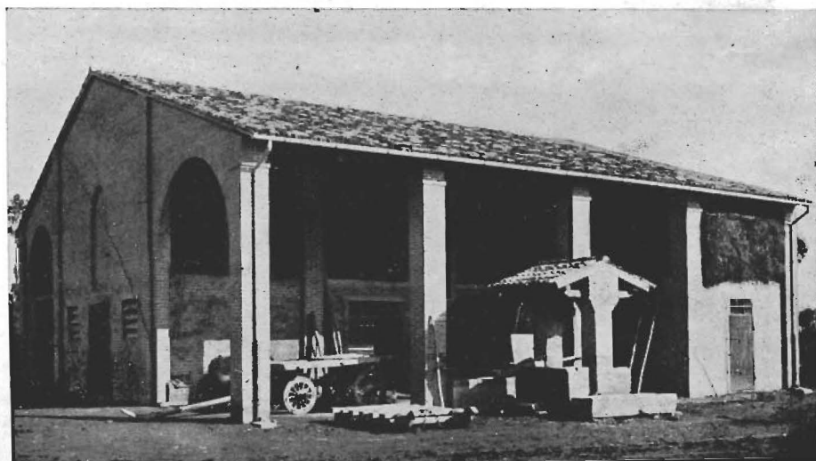
Boaria per 25 capi (Bondeno)
