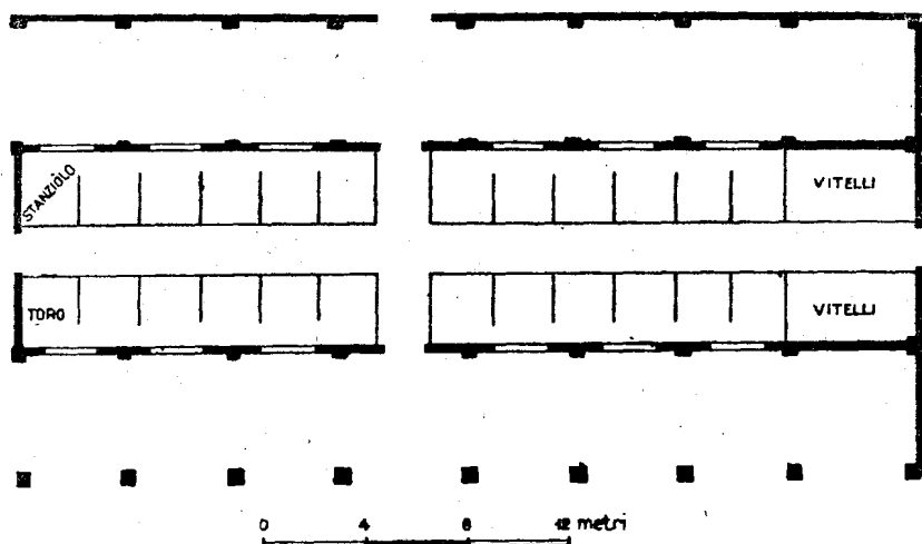
Pianta di una boaria per 50 capi
