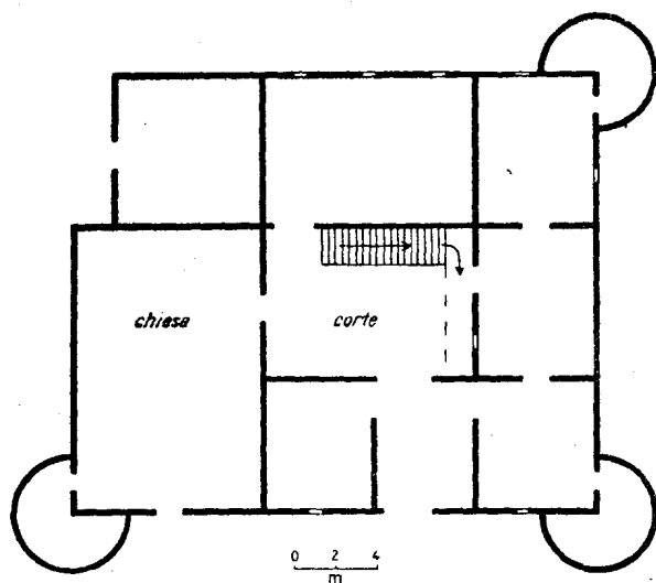
FIG. 4. - MASSERIA FORTIFICATA A MACCHIA. (Planimetria del piano terreno).
